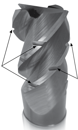
Detail přerušovaného břitu - obvodové drážky ve spirále
