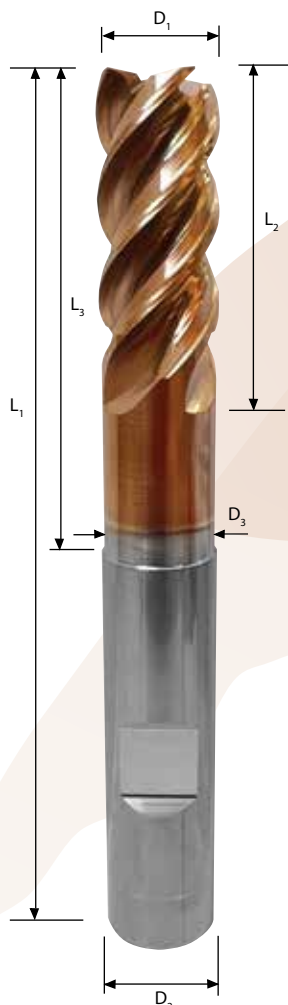
Detail břitu
