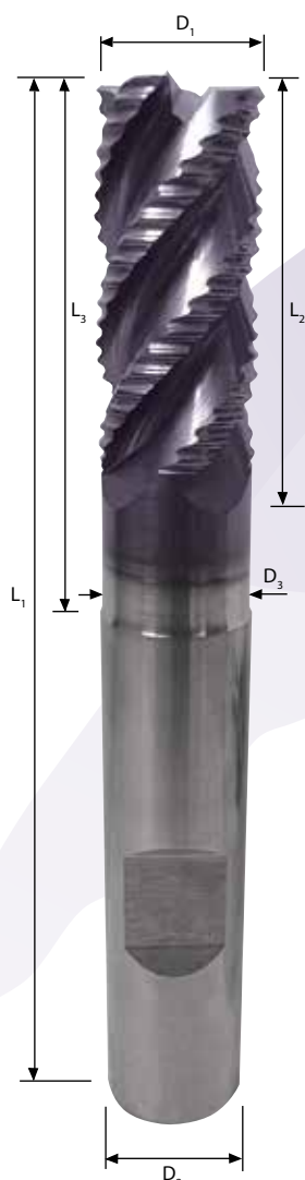
Detail břitu
