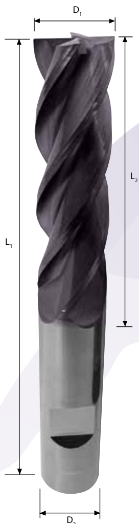
Detail břitu
