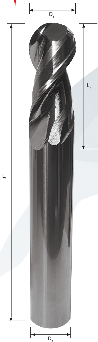
Detail břitu
